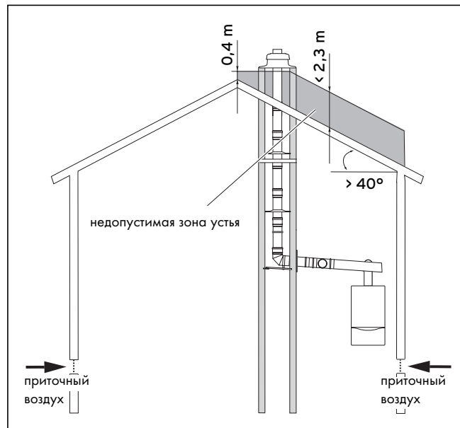
Рис. 2.1 Недопустимая область устья при наклоне крыши > 40°; независимо от положения отверстий приточного воздуха
