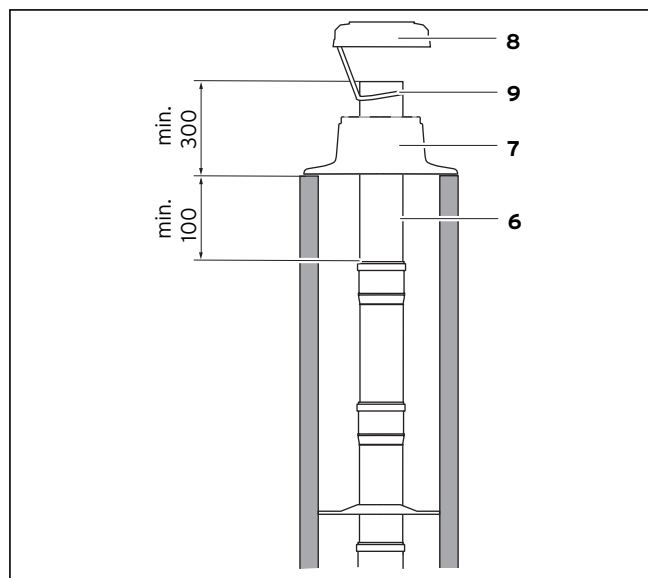
Obr. 4.7 Montáž potrubí pro odvod spalín
