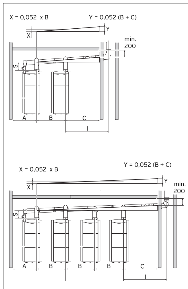
Obr. 4.4 Rozmery v priestore inštalácie plynových kompaktných zariadení s výhrevnou technikou a plynovým výhrevným kotlom
