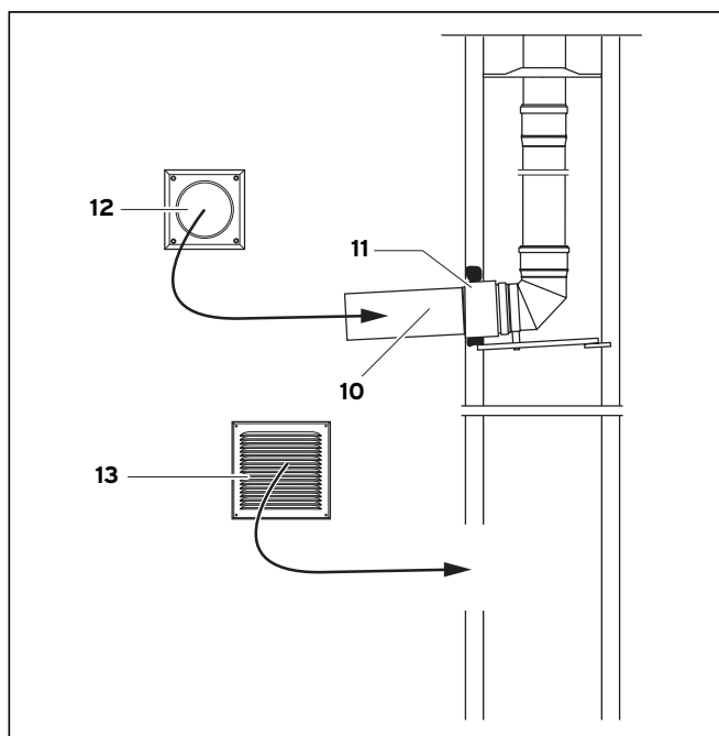
Obr.4.8 Namontujte rúru na odvod spalín, ochrannú rúru, tienidlo muriva a vetraciu mriežku
