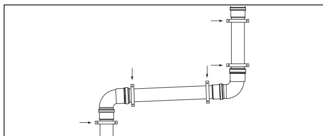
Obr. 4.18 Montáž spôn podľa presmerovaní
