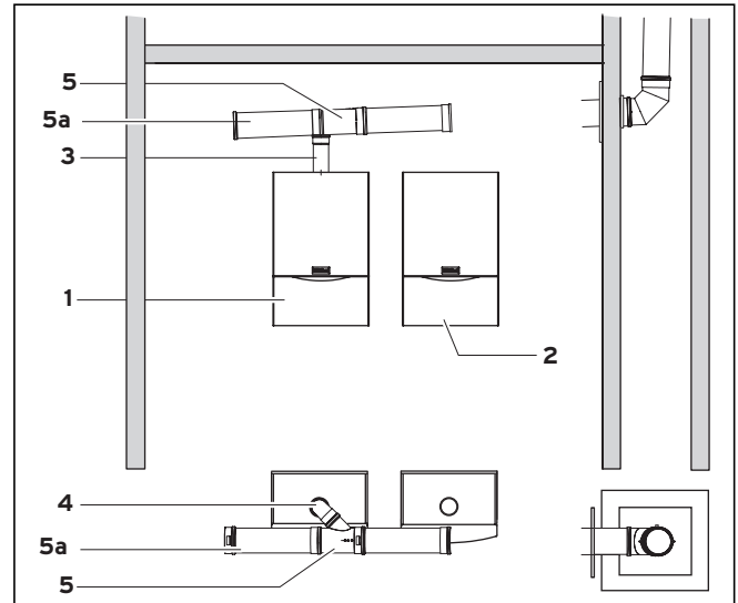
Мал. 4.9 Монтаж основного комплекту 00 2004 2761
