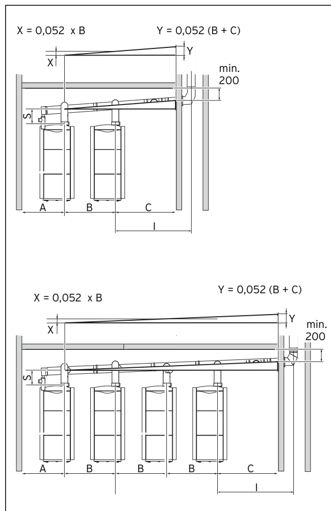
Мал. 4.4 Розміри у приміщенні установки компактного конденсаційного газового опалювального приладу та газового конденсаційного котла
