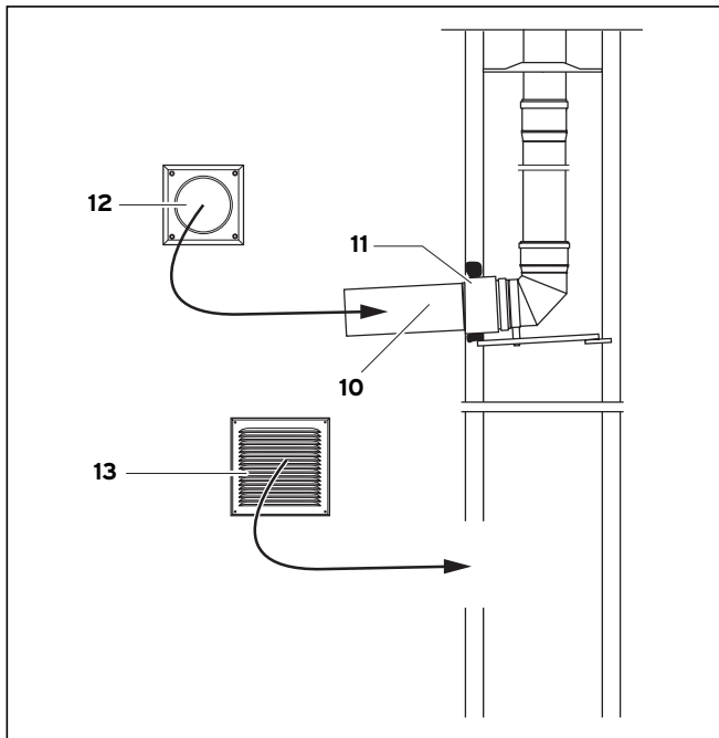
Мал. 4.8 Установка трубы газовідводу, опірної труби, стінної заглушки та вентиляційної решітки
