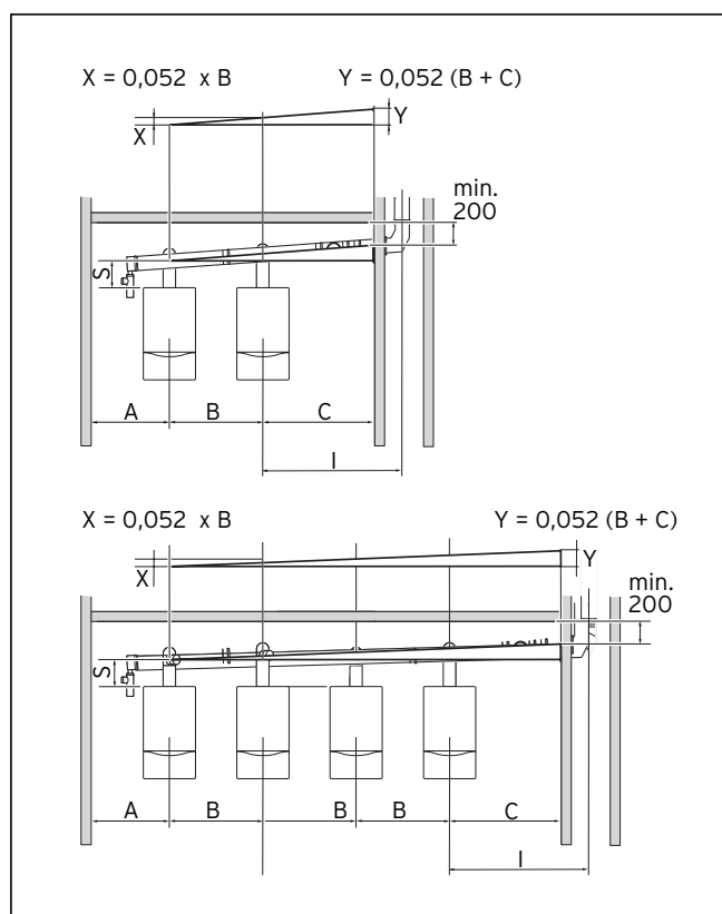
Мал. 4.2 Розміри у приміщенні установки конденсаційних настінних газових опалювальних приладів
