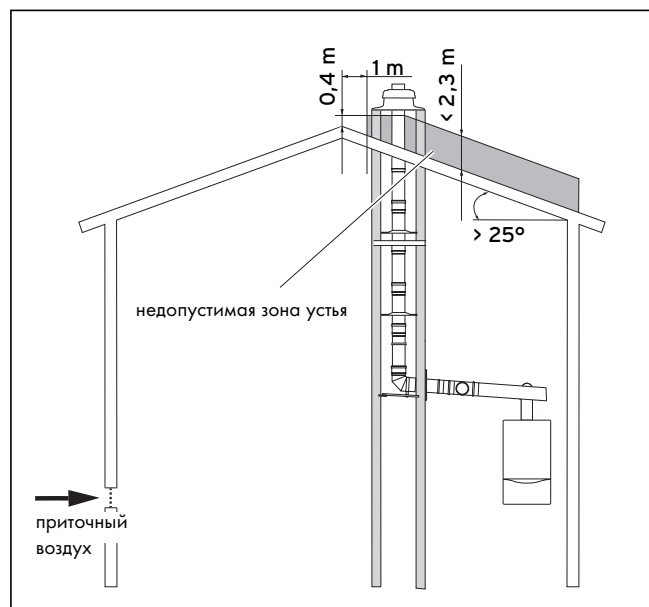
Рис. 2.2 Недопустимая область устья при наклоне крыши > 25°, но только в том случае, если отверстия приточного воздуха и шахта находятся на противоположных сторонах от конька крыши
