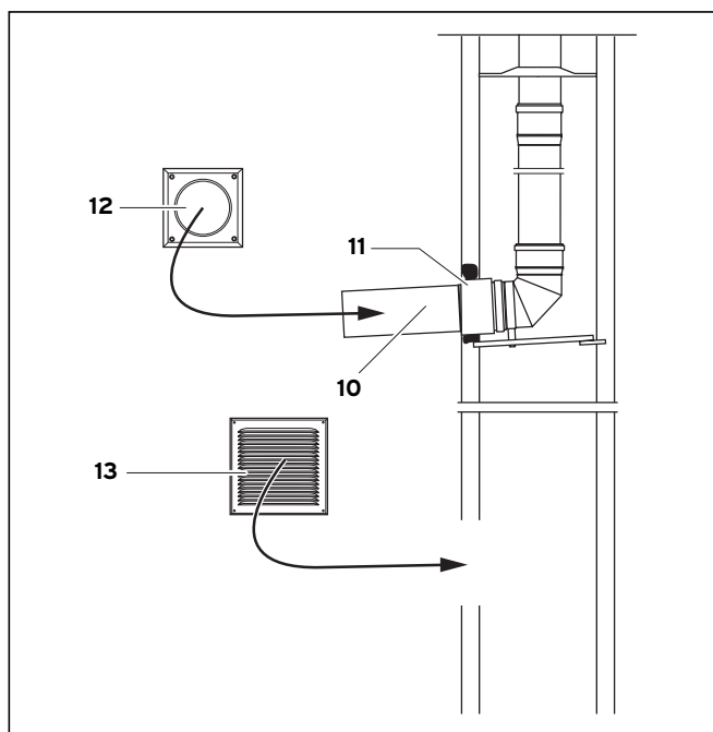
Рис. 4.8 Монтаж трубы газоотвода, защитной трубы, заглушки и вентиляционной решетки
